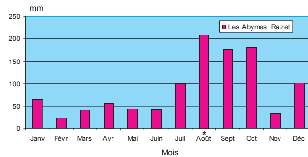
Pluviométrie au Raizet en 2007
